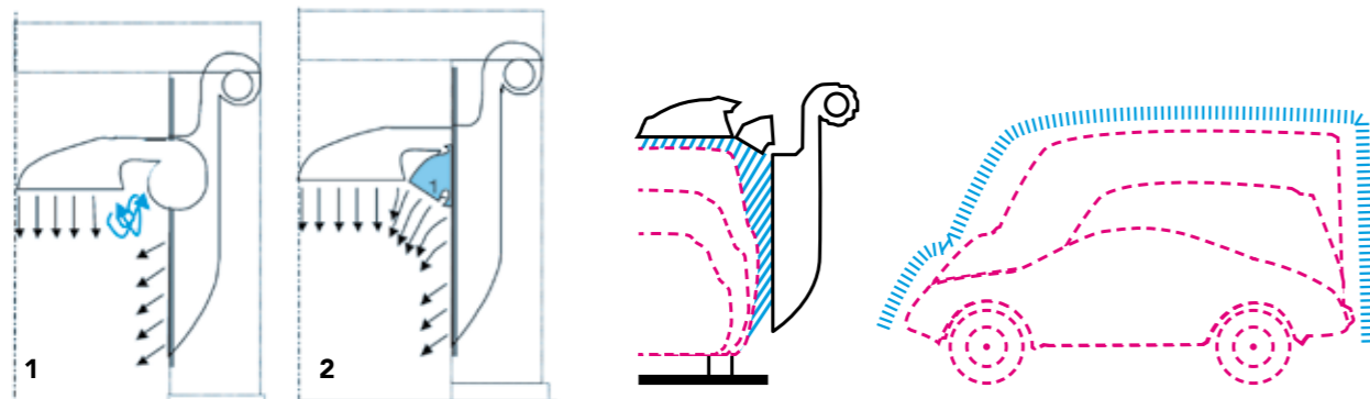
1 flussi d'aria senza convogliatore
